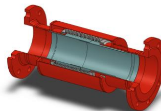
DN80-350 kołnierze sztykowe
