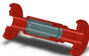
DN20-65 Kołnierze sztykowe
