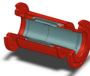
DN80-350 kołnierze płaskie
